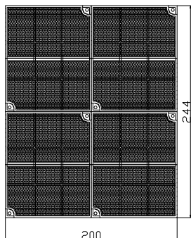
图 11b 四块反射器安装示意图（图未按比例）
