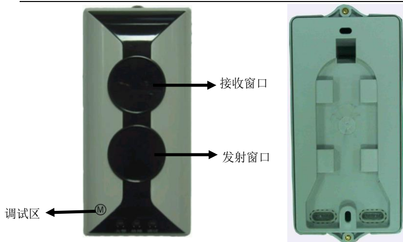
图 1 探测器外形示意图
