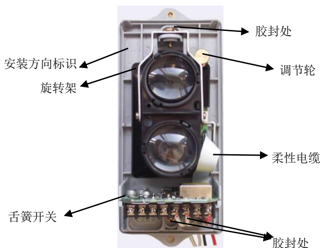
图 2 内部器件及胶封示意图
